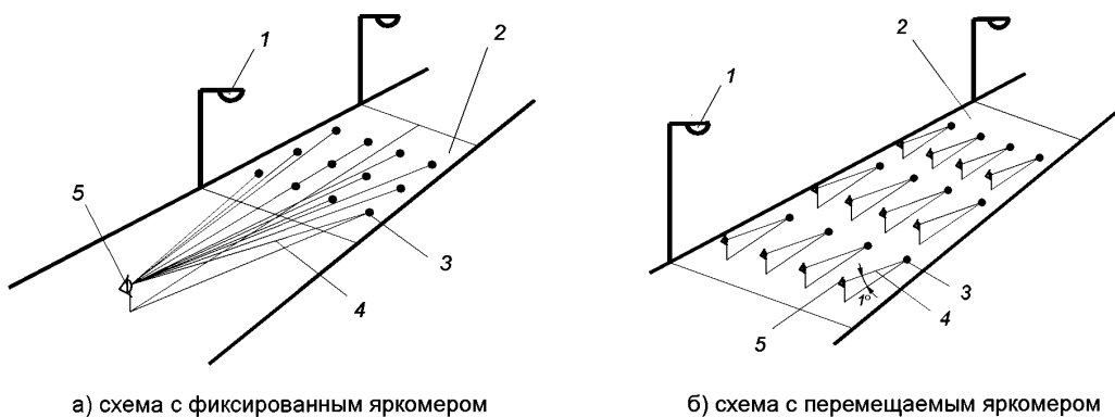
1 – ОП; 2 – контрольный участок; 3 – точка измерения; 4 – оптическая ось; 5 – яркомер
